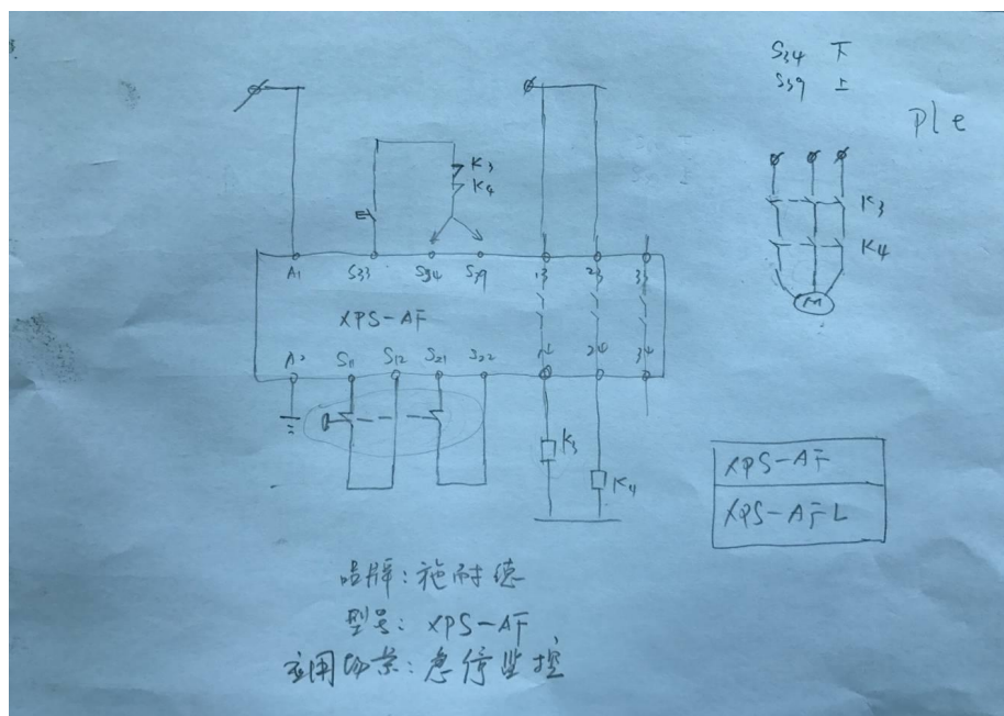
上图是施耐德 Schneider-XPS-AF5130 安全继电器接线在急停应用场景中的接线图
