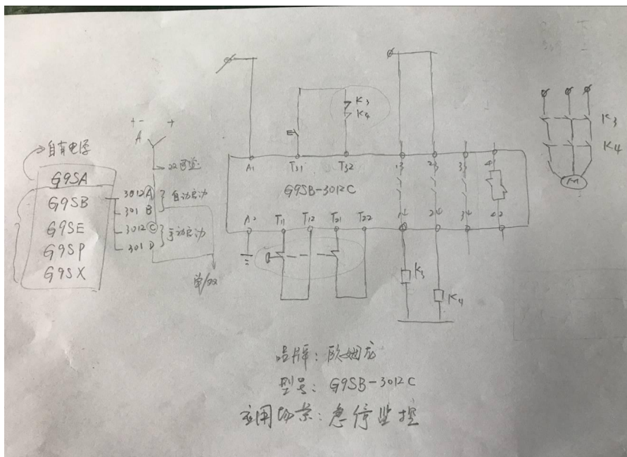
上图是 欧姆龙 OMRON 安全继电器在急停应用场景中的接线图
